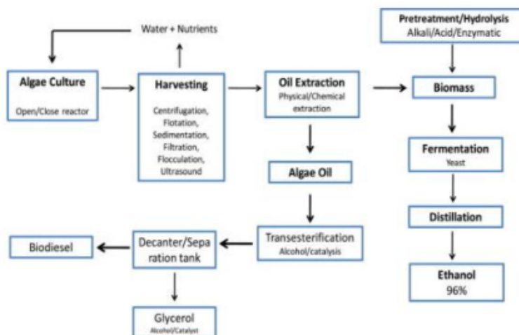
Gambar 3.33. Produksi biodiesel dan bioethanol dari mikroalga
