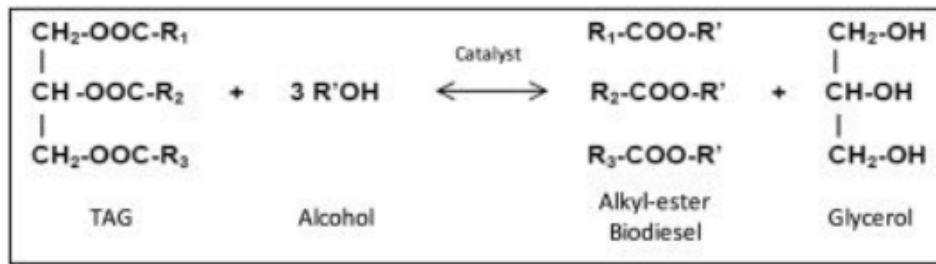
Gambar 3.32. Reaksi tranesterifikasi
