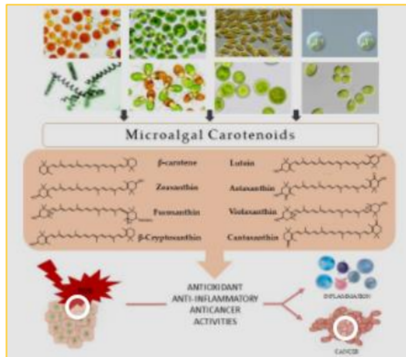
Gambar 3.35. Karotenoid mikroalga dan manfaatnya.
