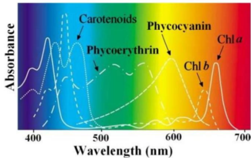
Gambar 3.5. Beberapa pigmen dari mikroalga
