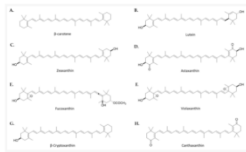
Gambar 3.36. struktur kimia kelompok karotenoid
