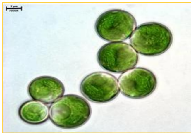
Gambar 3.38. Parietochloris alveolaris (mikroalga hijau)
