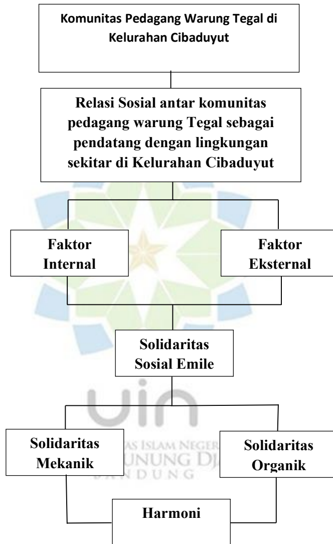
Gambar 1.1. Skema Berpikir
