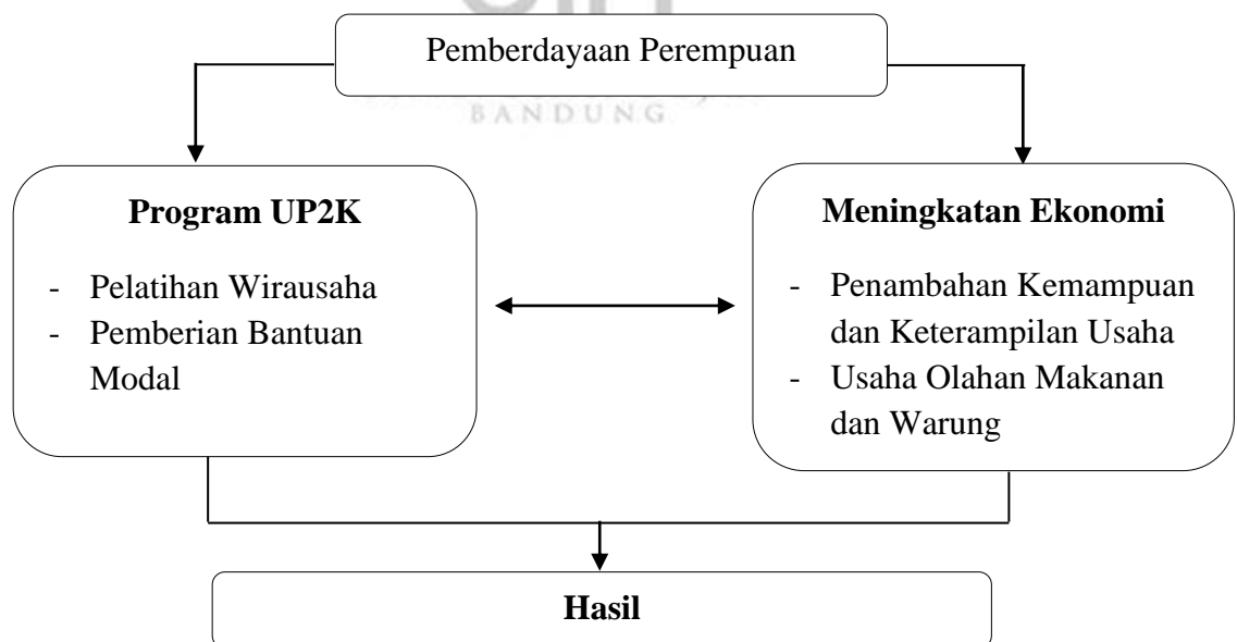
Gambar 1.1 Kerangka Konseptual
