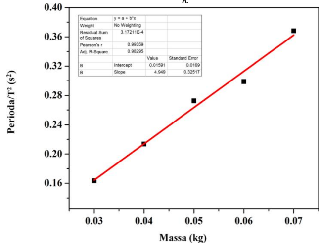
Gbr. 6 Grafik massa ( m ) terhadap perioda ( T^2 ) dengan variasi massa: 30-gr, 40-gr, 50-gr, 60-gr dan 70-gr.
