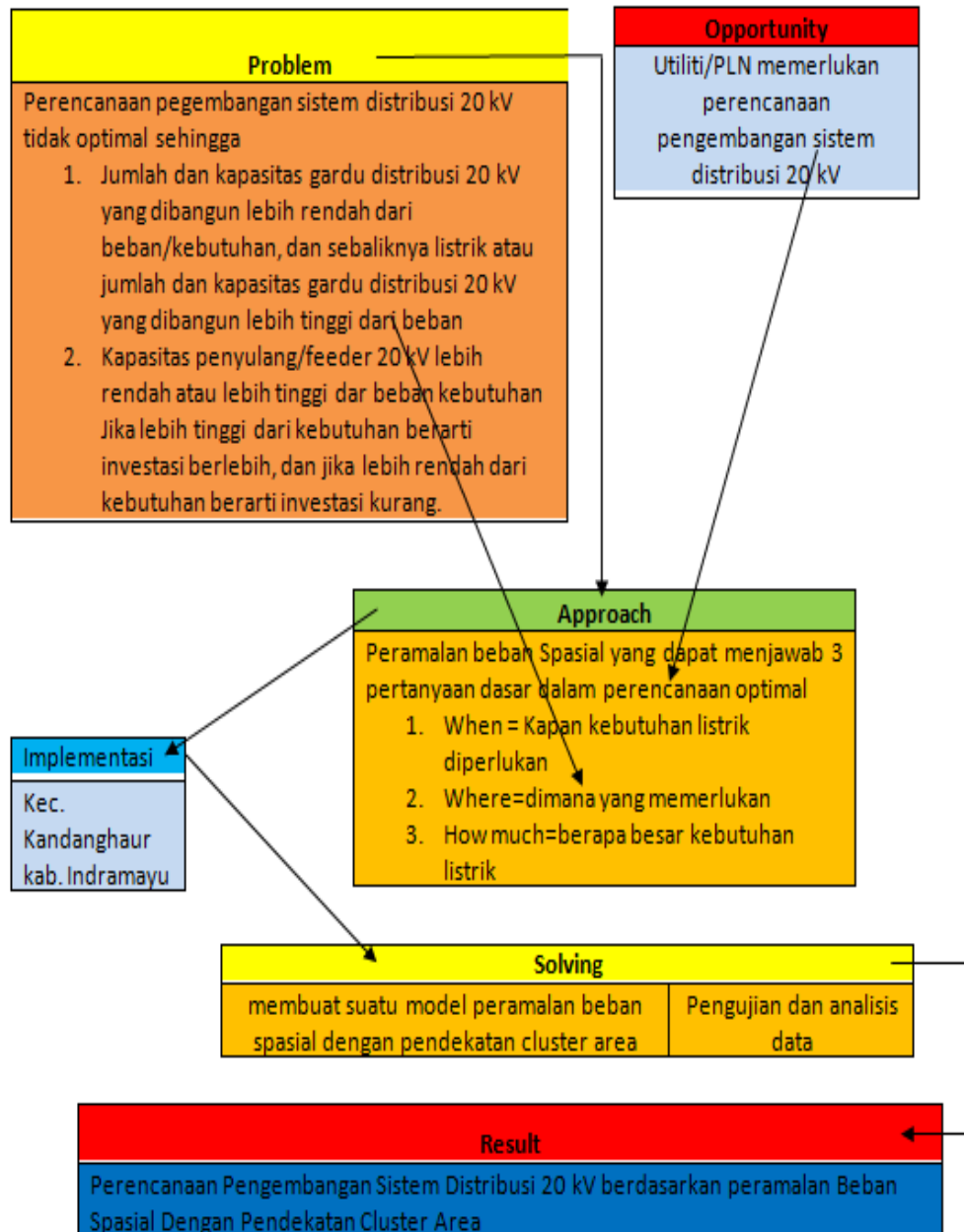
Gambar 1.1. Kerangka Berfikir
